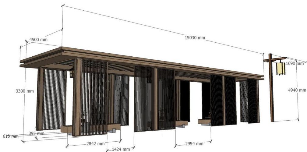
图 5-54 街道亭尺寸图
