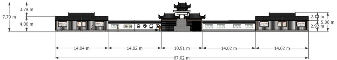
图 5-27 文化长廊主视图
