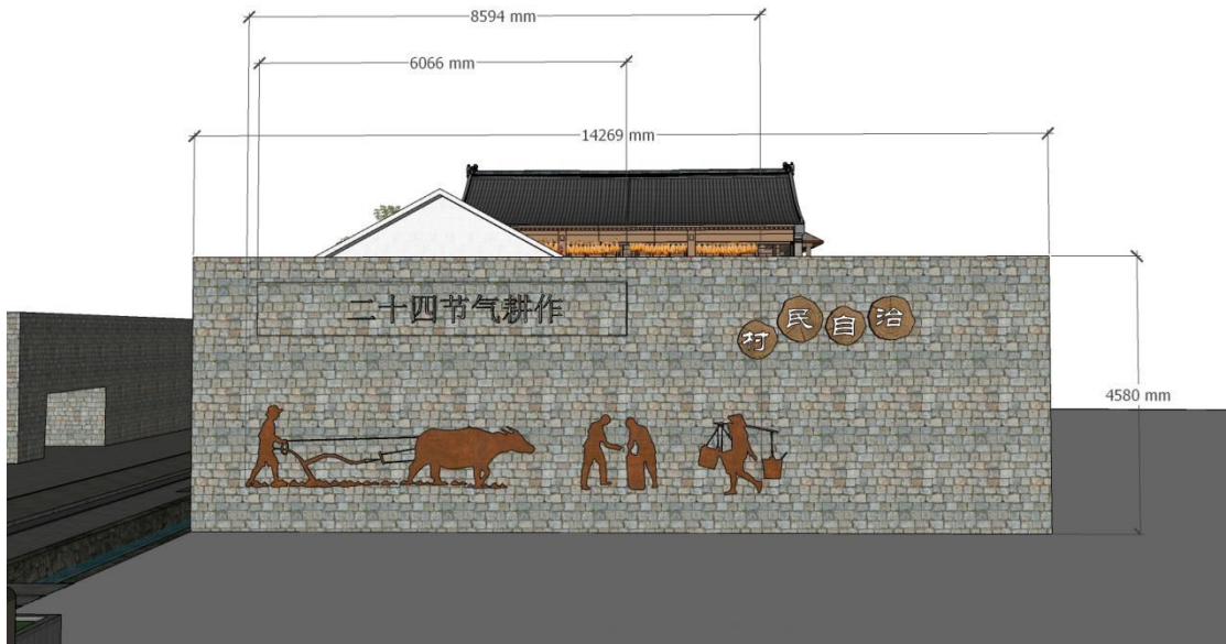
图 5-57 背景墙尺寸图
