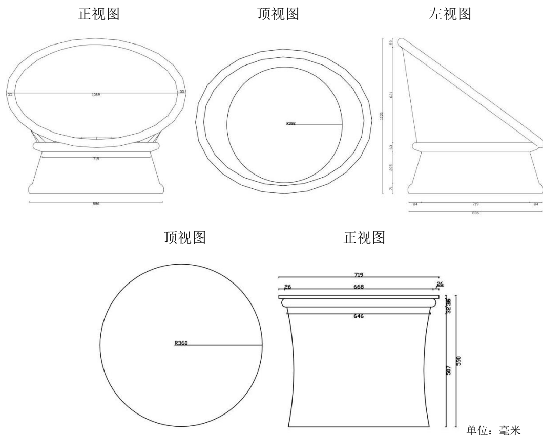
图 5-25 竹编桌椅三视图
