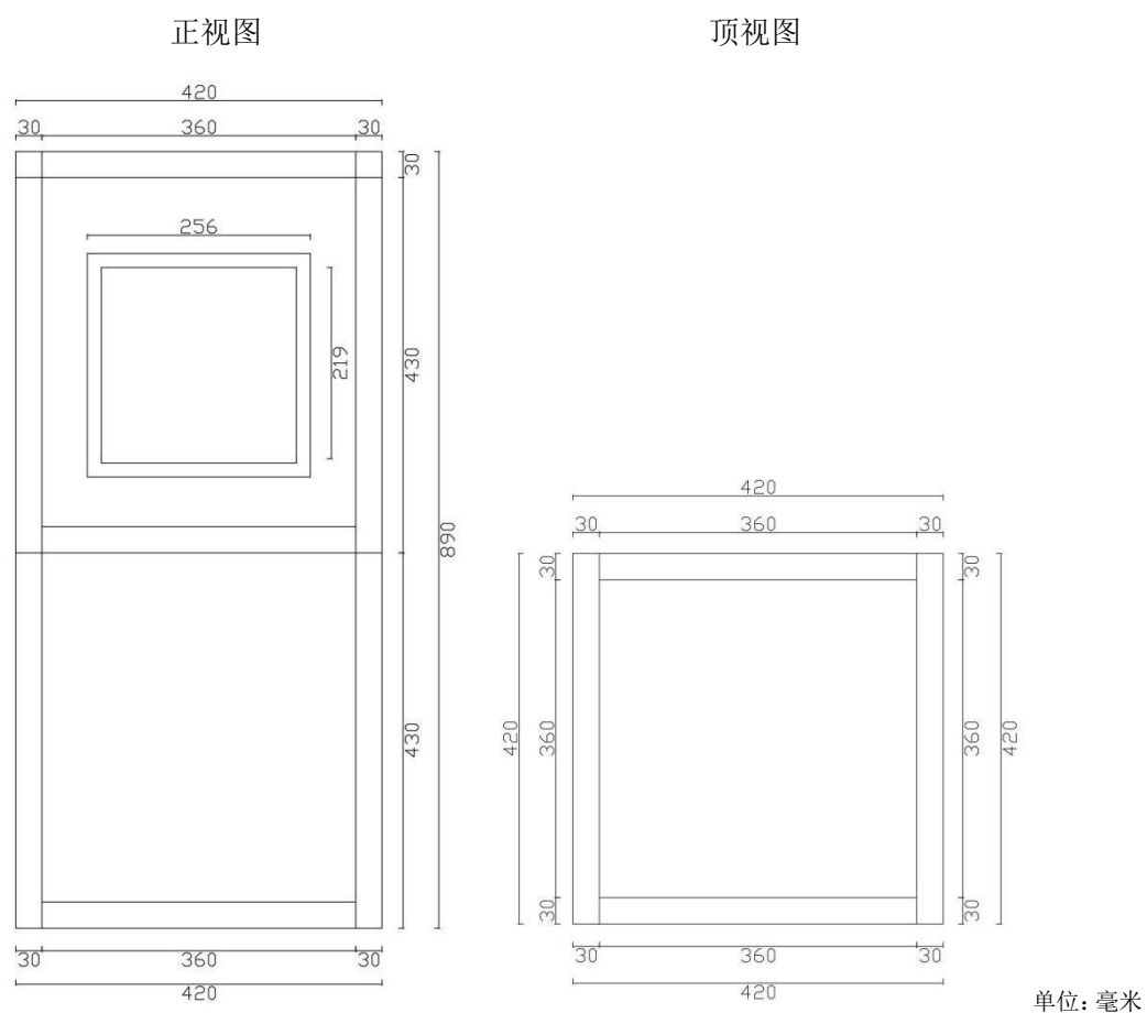
图 5-23 垃圾桶正视图与顶视图
