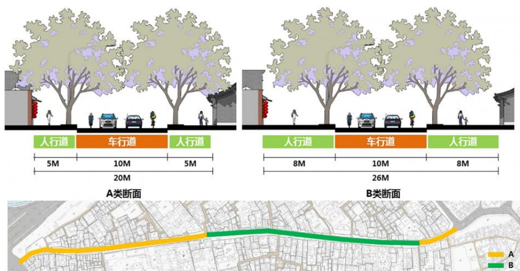
图 2-5 道路断面分析图
